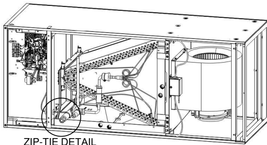
ZIP-TIE DETAIL
