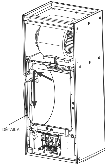
Le faisceau de câblage
