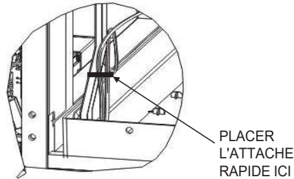
DETAILS DE L'ATTACHE RAPIDE
