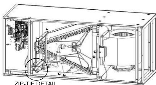
ZIP-TIE DETAIL
