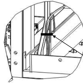
ZIP-TIE DETAIL
