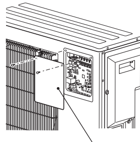
Panneau d'entretien
