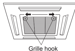
Grille hook
